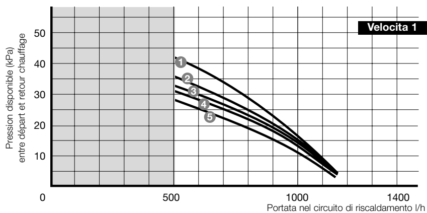
Curva portata/pressione disponibile Themafast C 30 E e F 30 H-MOD
