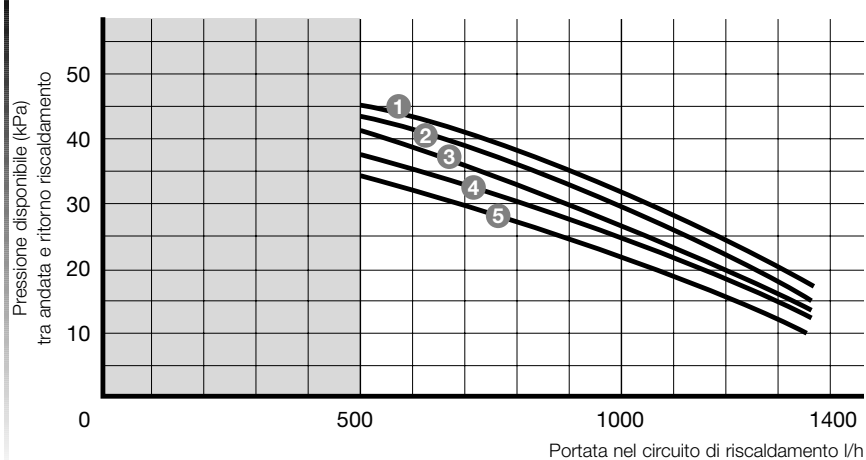
Curva portata/pressione disponibile Themafast C 24 E NOx e F 24 E NOx
