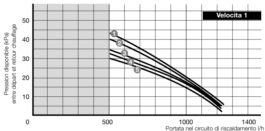
Curva portata/pressione disponibile Themafast C 25 E e F 25 H-MOD
