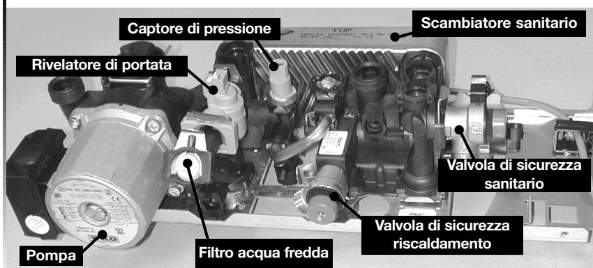
Blocco idraulico
