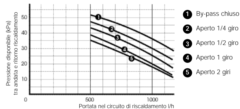
Curva portata/pressione disponibile
